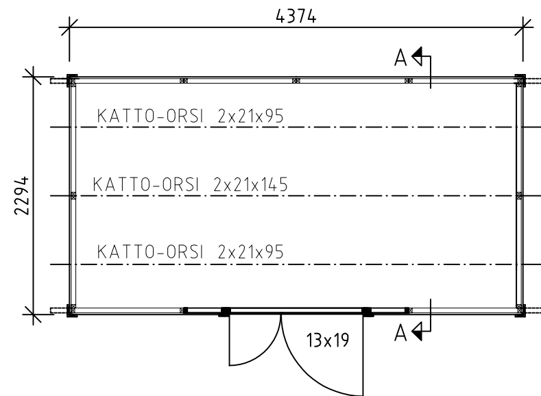
SUUNNITELMA
