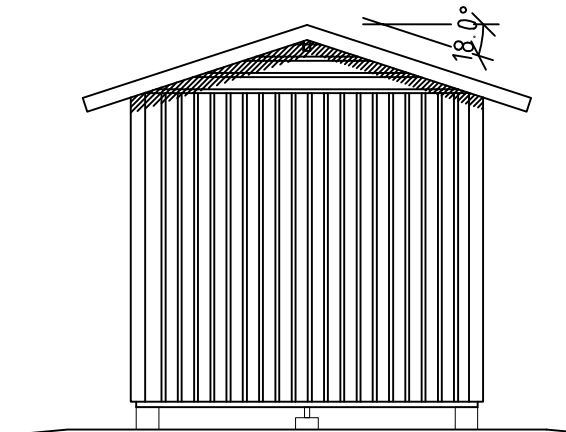
PÄÄTY, OIKEA
