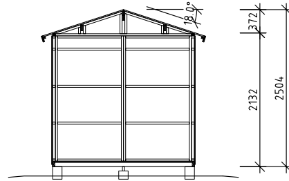
Läpileikkaus
