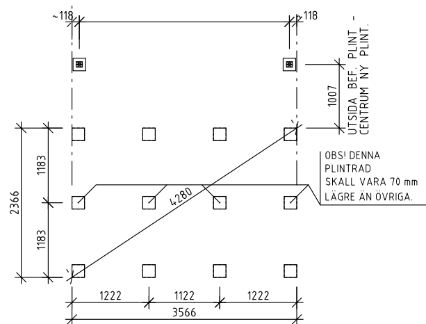
Perustuspiirustus
