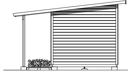
Pääty
