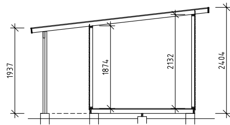
Läpileikkaus
