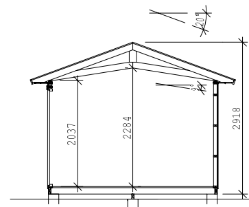
POIKKILEIKKAUS
