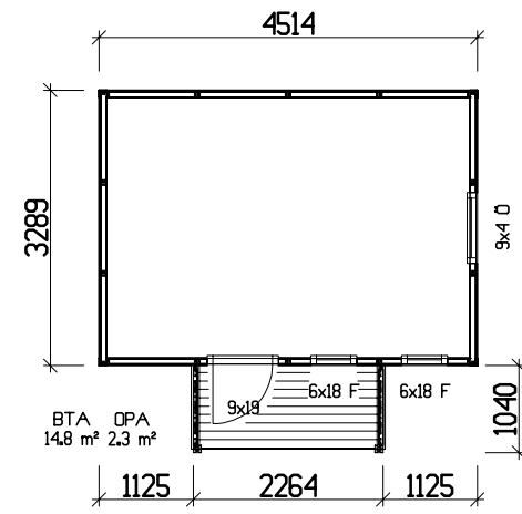
SUUNNITELMA
