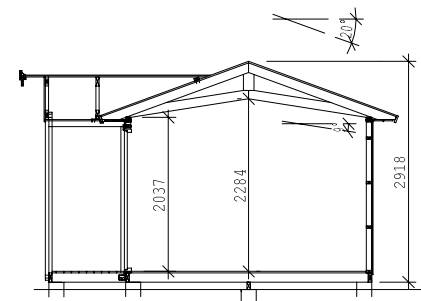
POIKKILEIKKAUS
