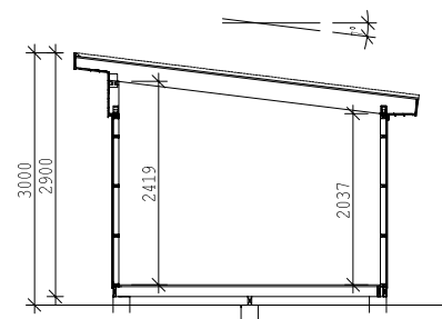
POIKKILEIKKAUS
