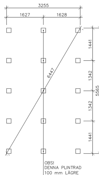
Perustuspiirustus
