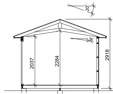
Läpileikkaus
