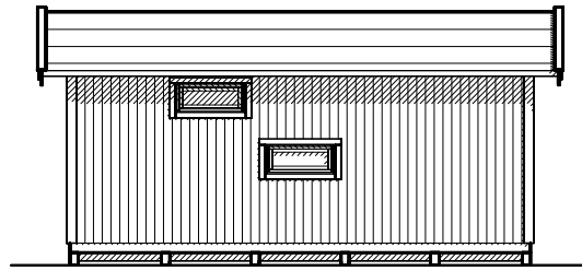
Pitkä sivu
