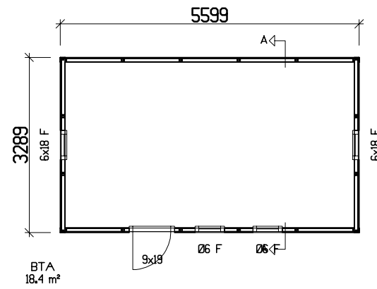
SUUNNITELMA
