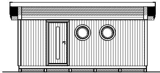
JULKISIVU
