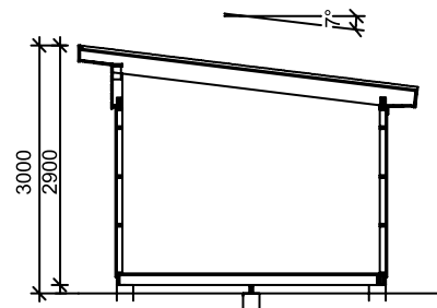
Läpileikkaus
