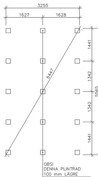
Perustuspiirustus
