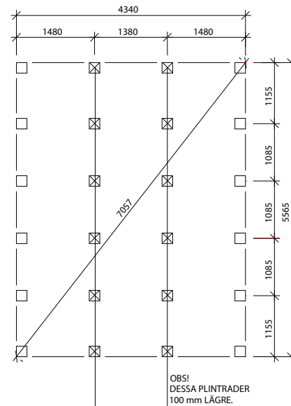
Perustuspiirustus
