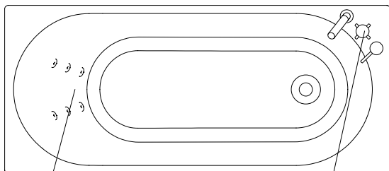
Selkähierontaosan sijoittaminen Kylpyammeen etulevy Tasoasennushanan paikka
