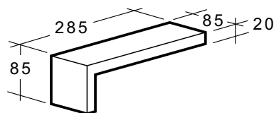
MTL ulkokulma 285/85
