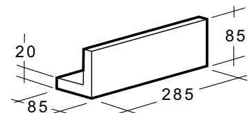
MTL yläkulma 285x85x85
